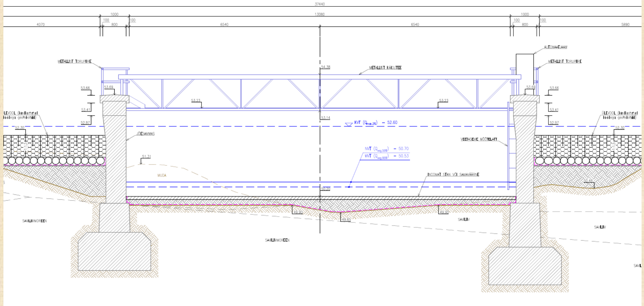
LÕIGE A-A
